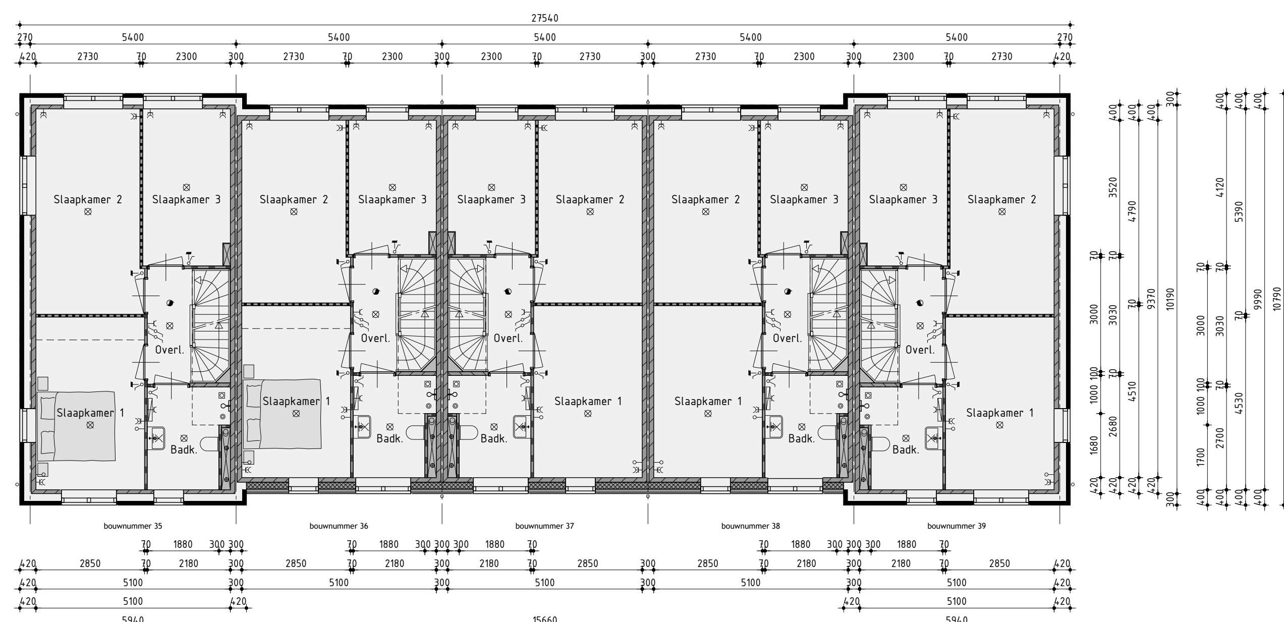
1ste verdieping
