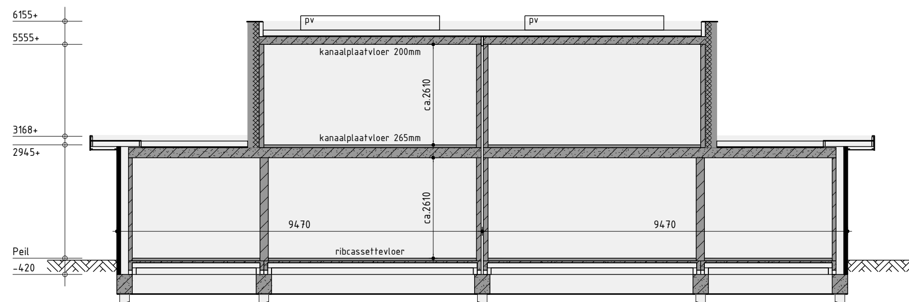
Principe doorsnede A-A
