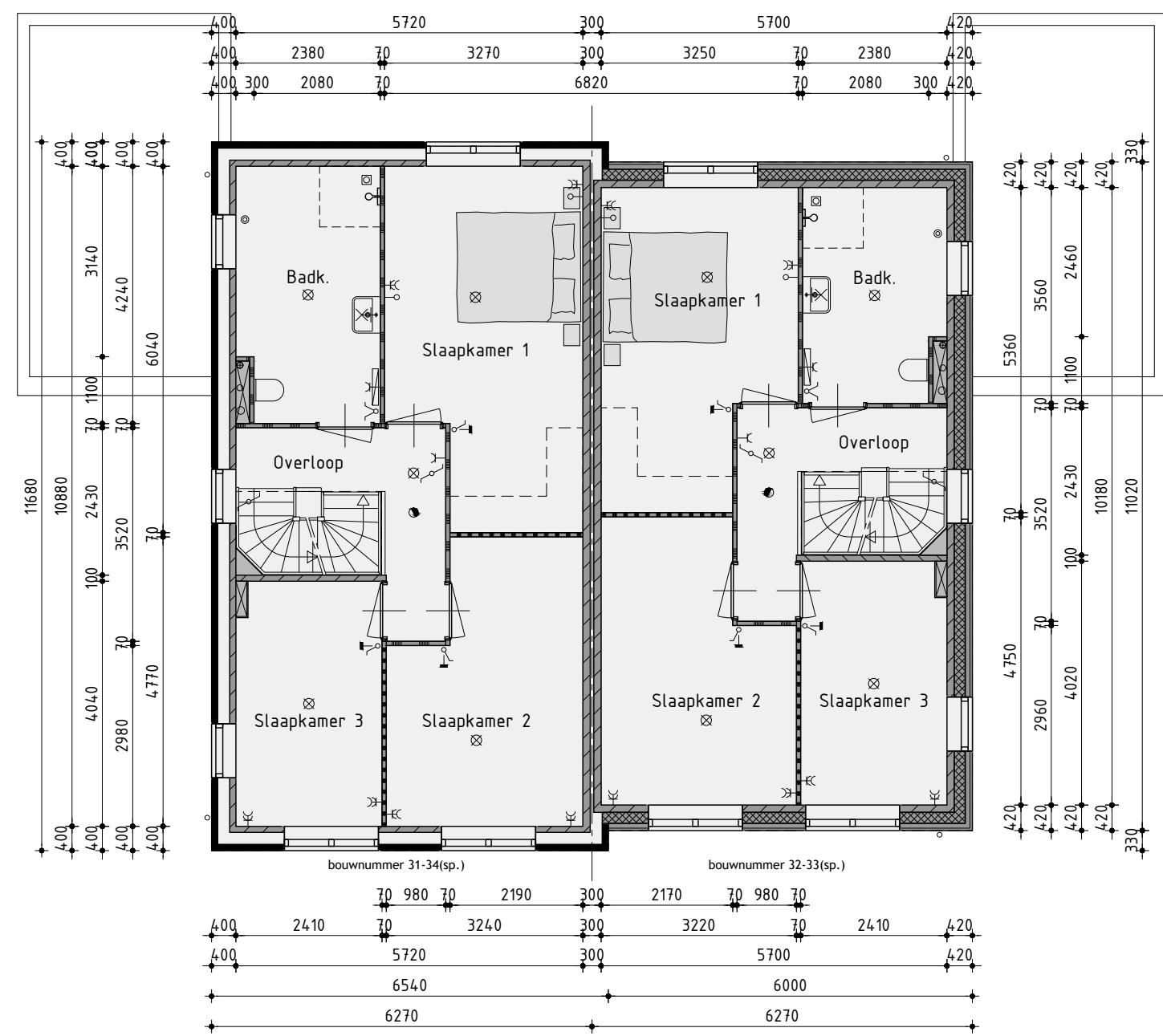
1ste Verdieping
