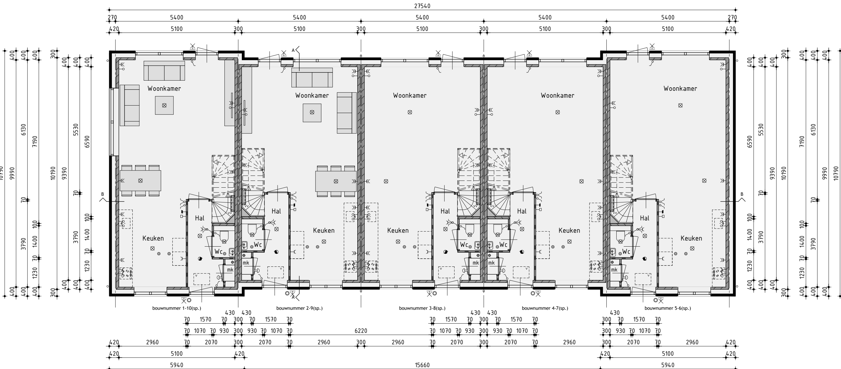
Begane grond
