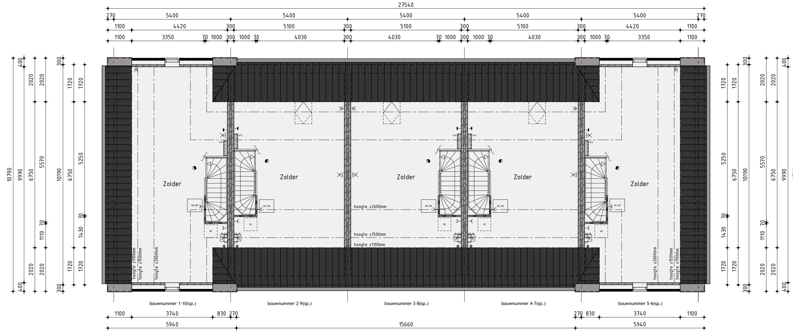
2de verdieping
