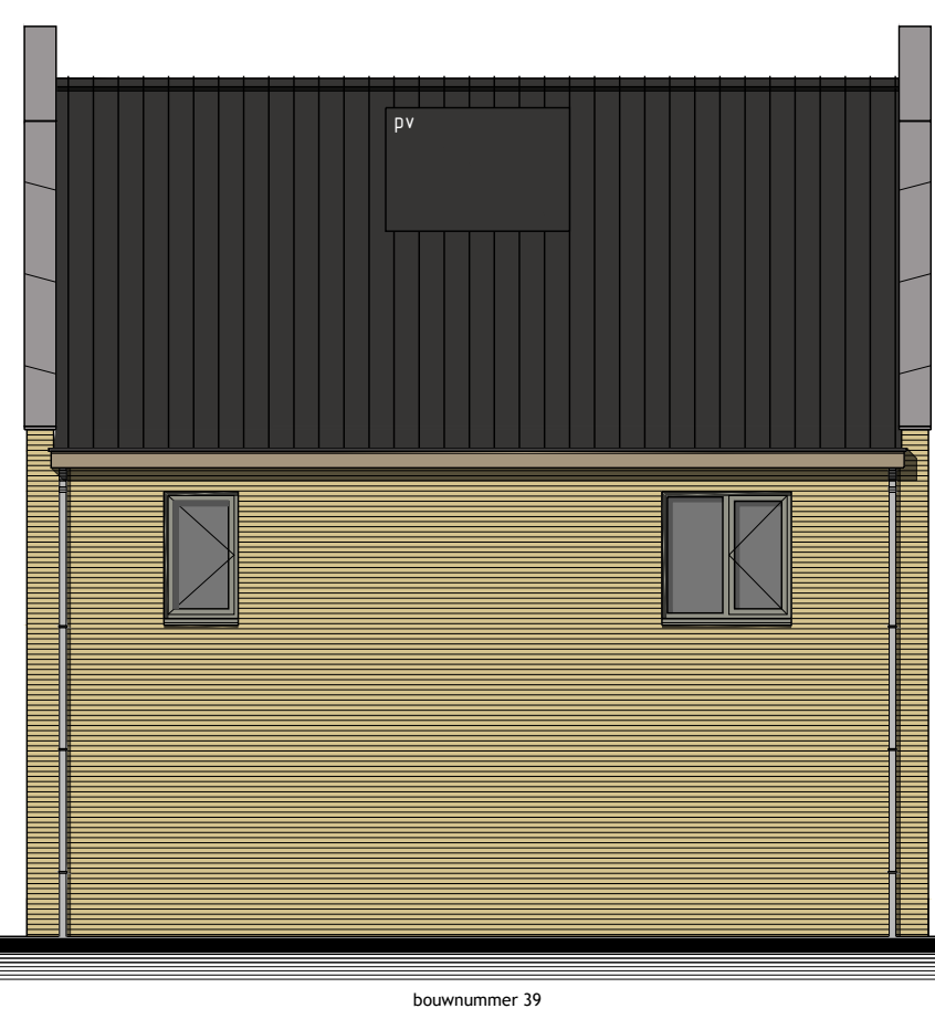
Rechter zijgevel
