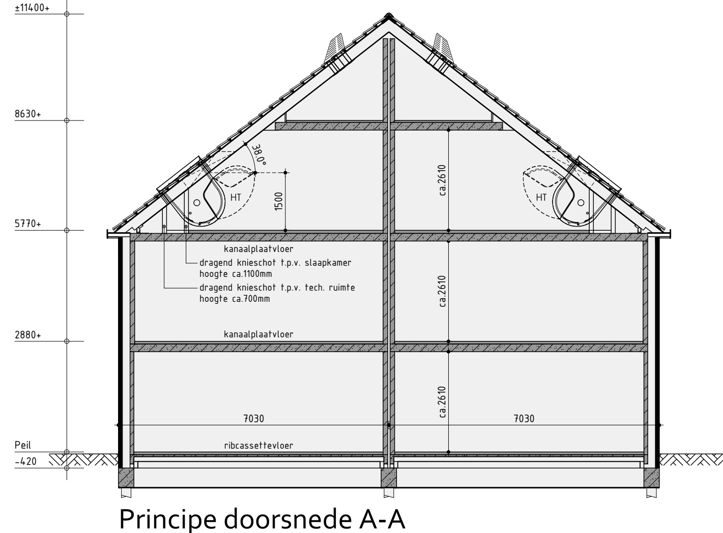
Principe doorsnede A-A
