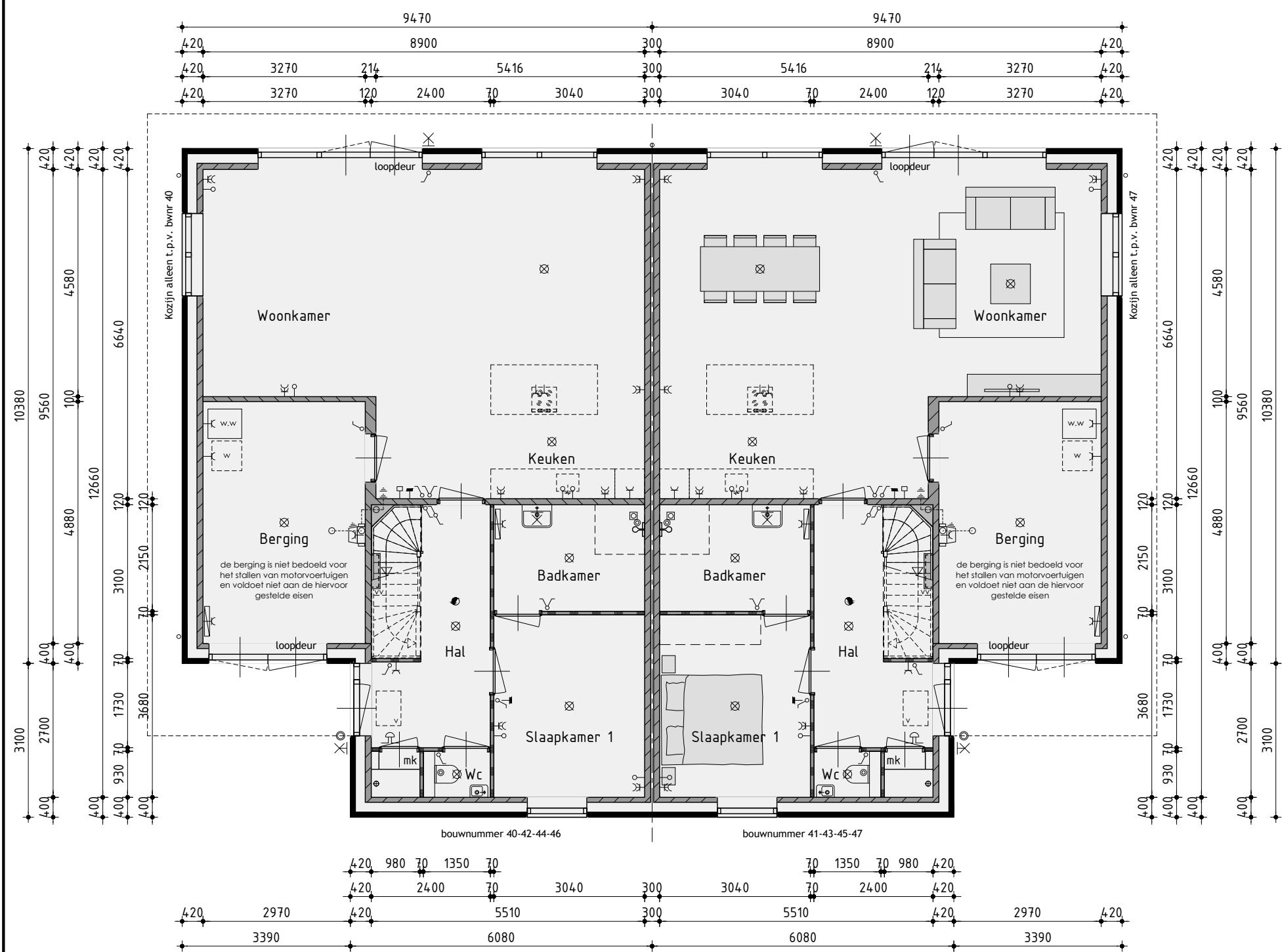
Begane grond
