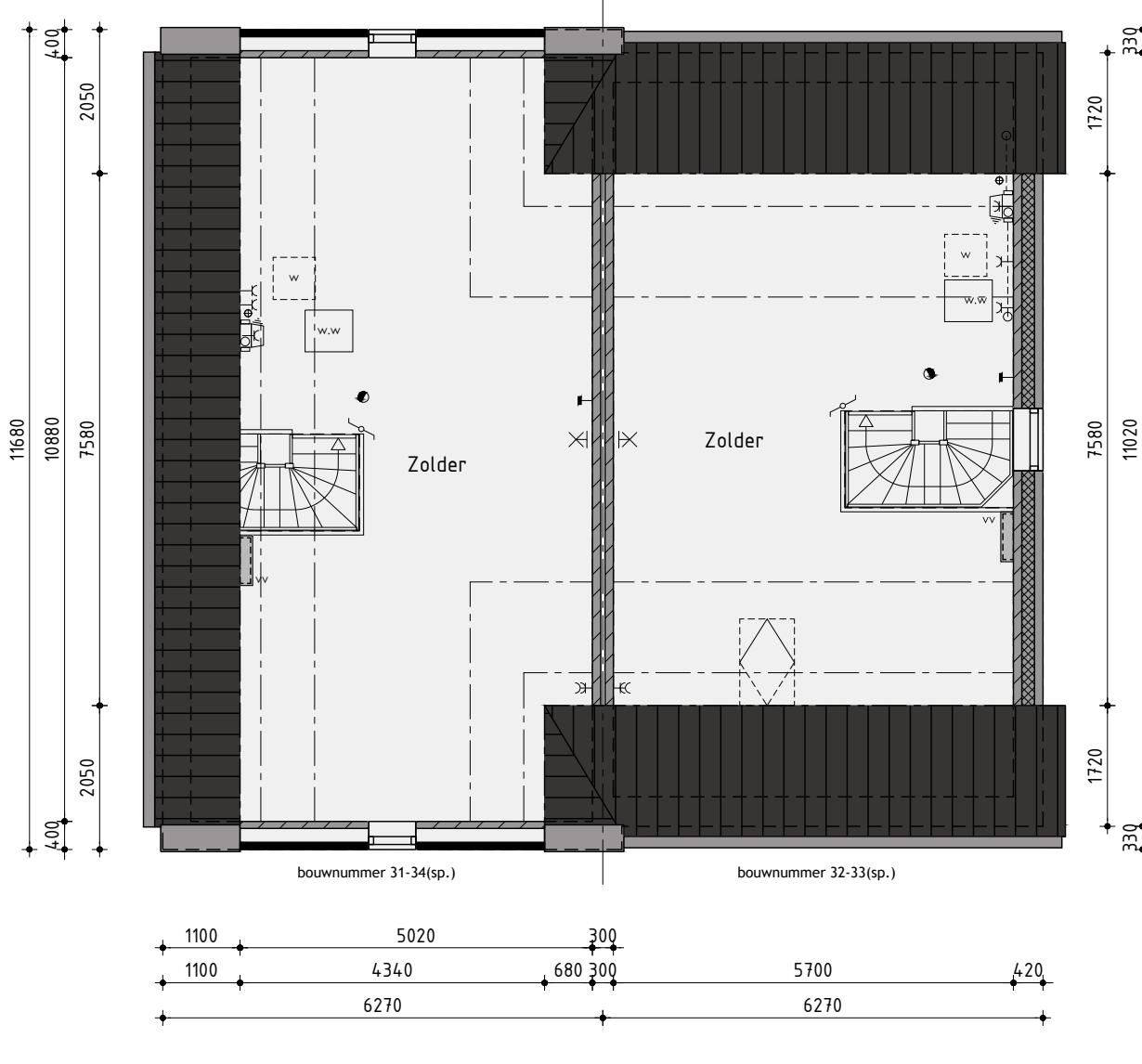
2de Verdieping
