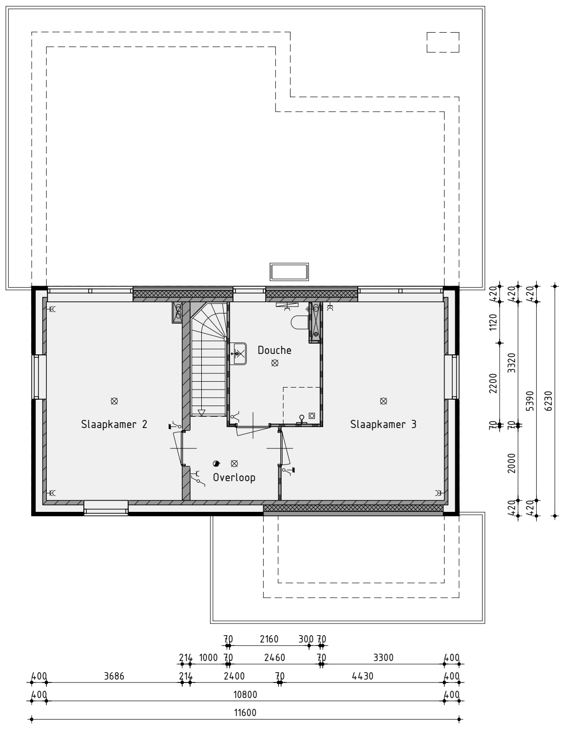
1ste Verdieping
