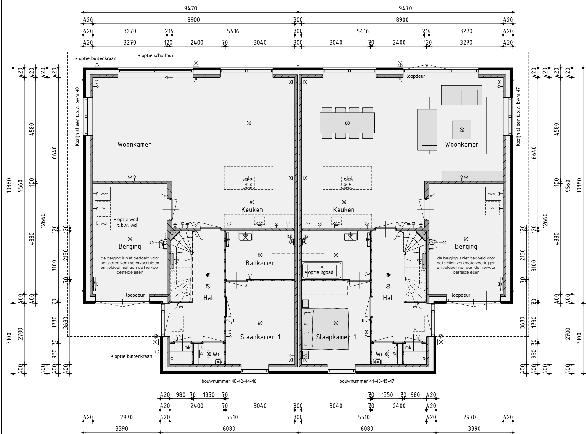
Begane grond
