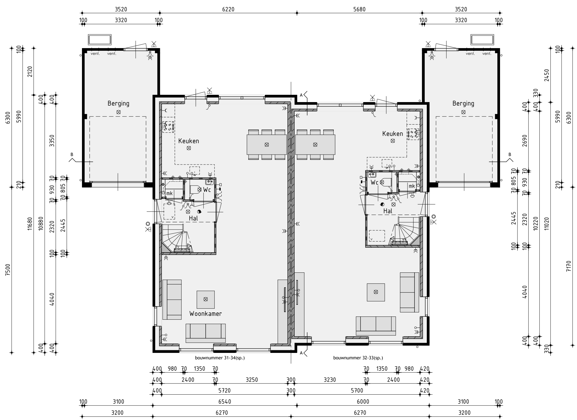
Begane grond
