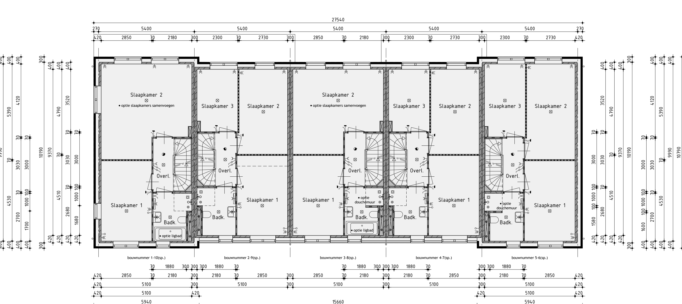
1ste verdieping v.z.v. vloerverwarming
