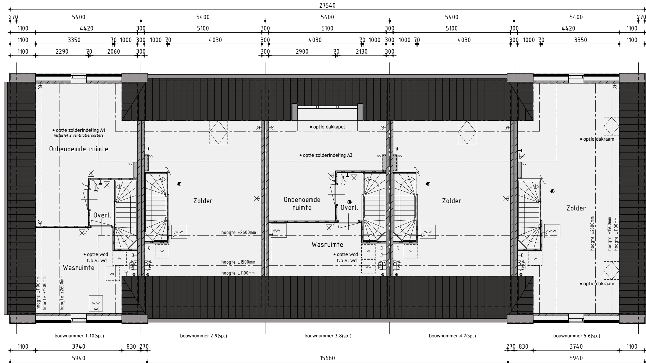
2de verdieping v.z.v. vloerverwarming
